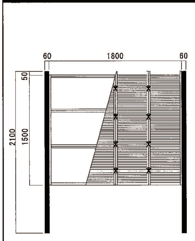
造作H1500mm 参考寸法図
