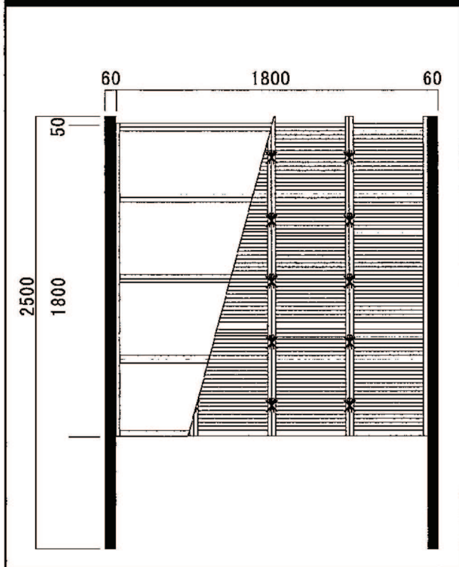
造作H1800mm 参考寸法図
