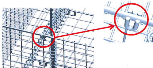
⑥上フタ面の受け金具を左右面前後面にはめ込んだ状態
